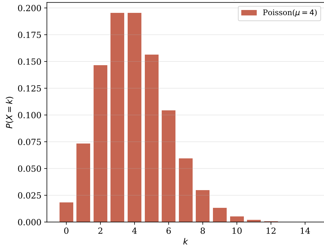
Diskrete Poisson-Verteilung (PMF)
