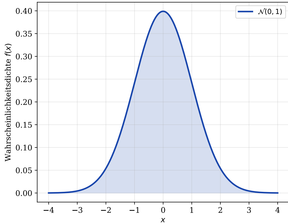
Kontinuierliche Normalverteilung (PDF)
