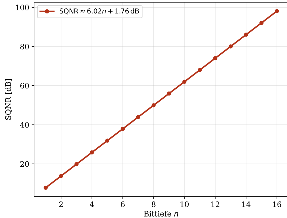
Quantisierungs-SNR vs. Bittiefe
