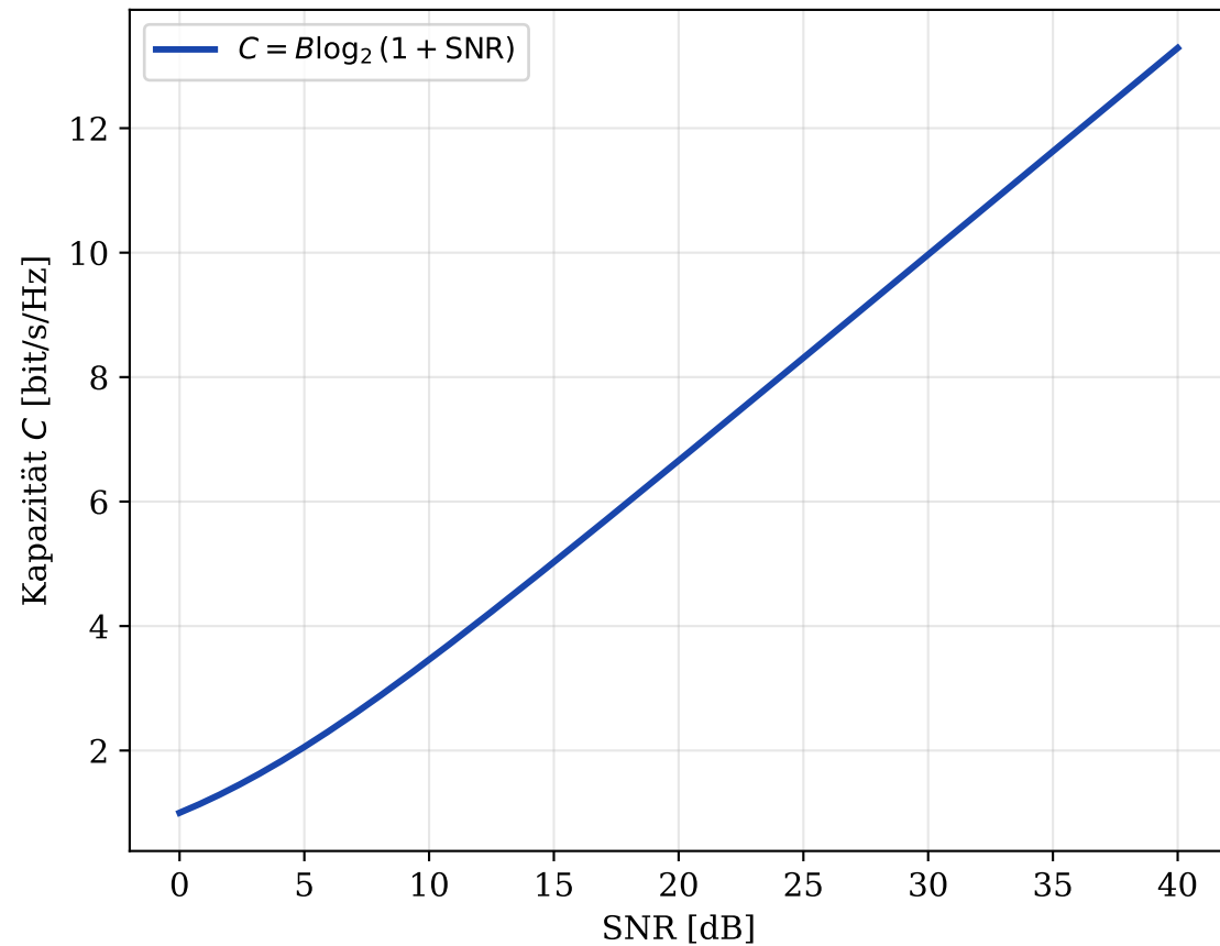
Shannon-Kanalkapazität ( B = 1 Hz)
