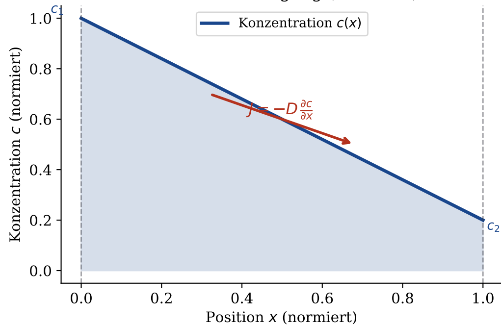
Membrandurchgang (stationär)
