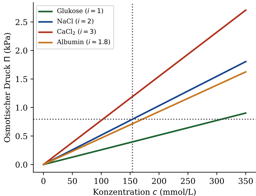
Osmotischer Druck vs. Konzentration
