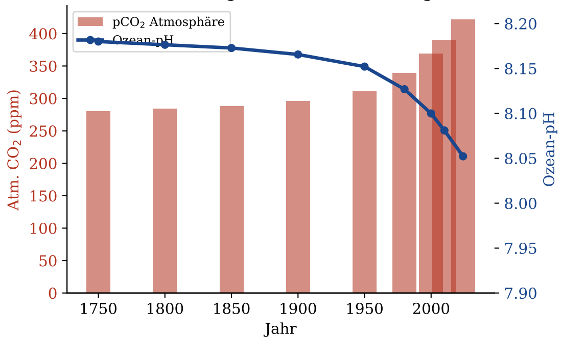
CO 2 -Anstieg & Ozeanversauerung
