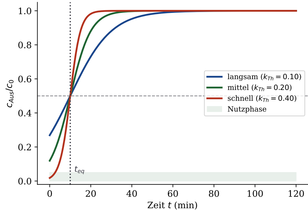
Durchbruchskurven (Thomas-Modell)
