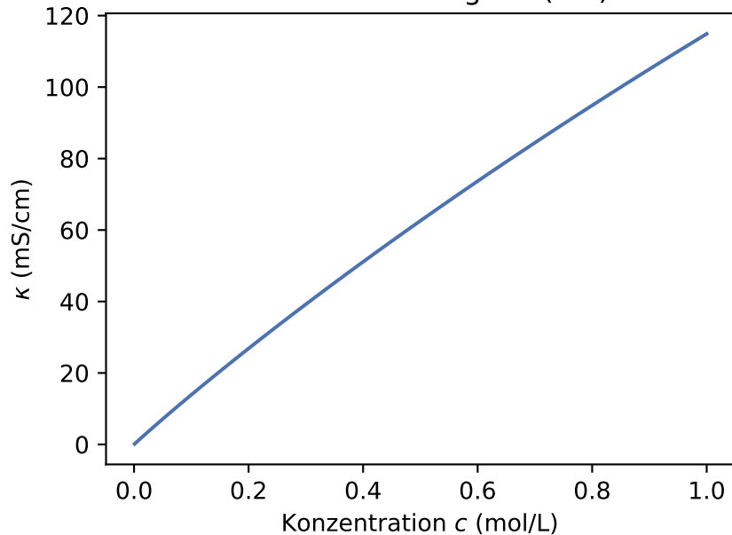
Ionische Leitfähigkeit (KCl)
