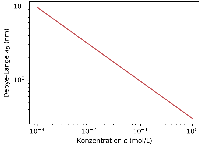
Debye-Längenskala
