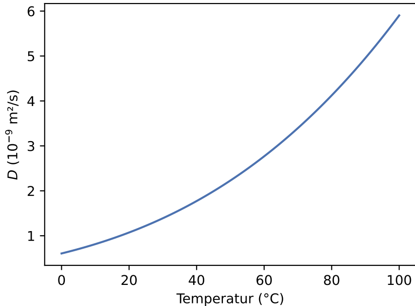
Einstein-Stokes-Diffusion
