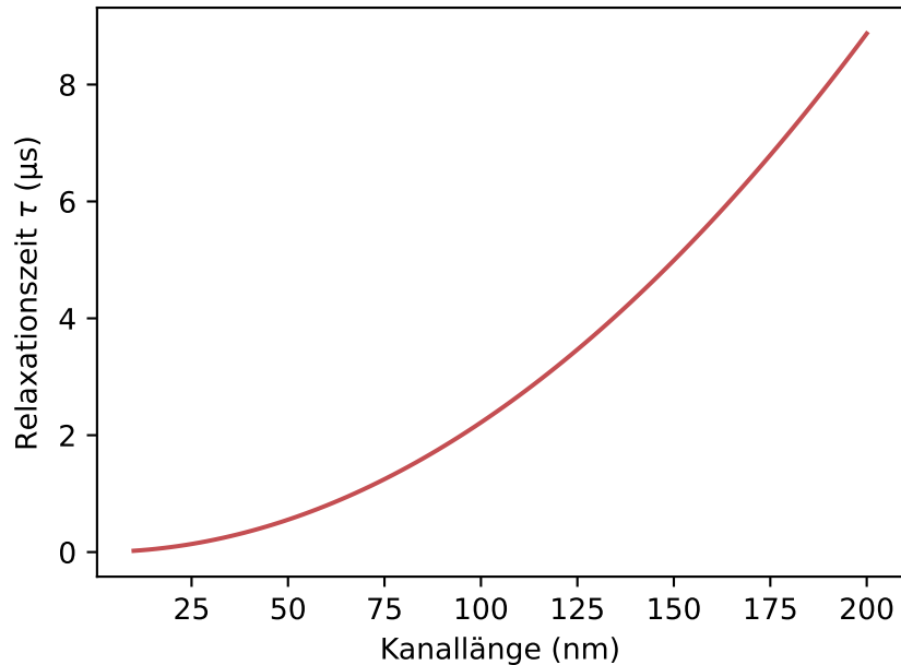
Relaxationszeit
