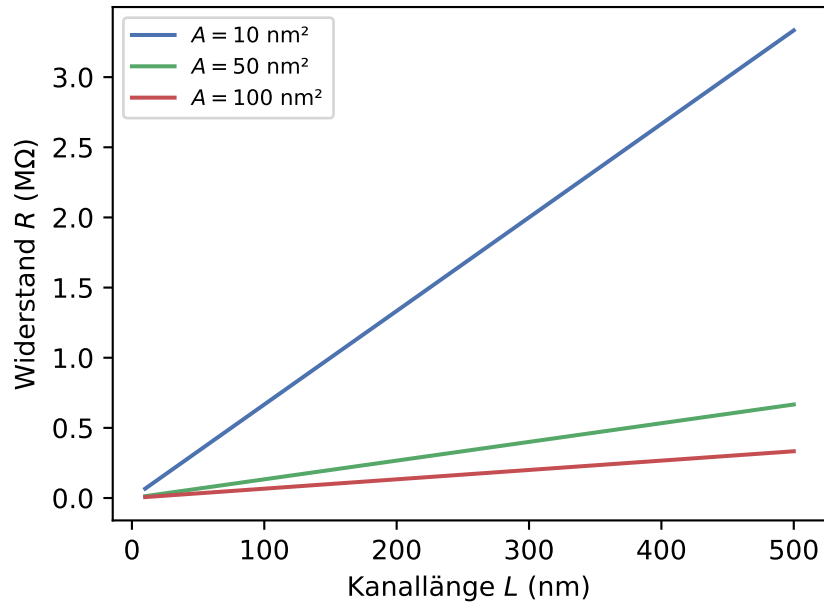
Widerstandsskalierung
