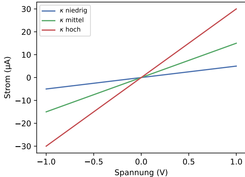
Ohmsches Verhalten
