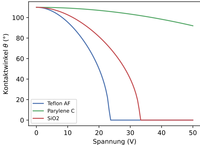
Young-Lippmann-Gleichung
