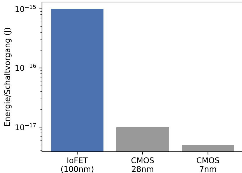
CMOS-Vergleich
