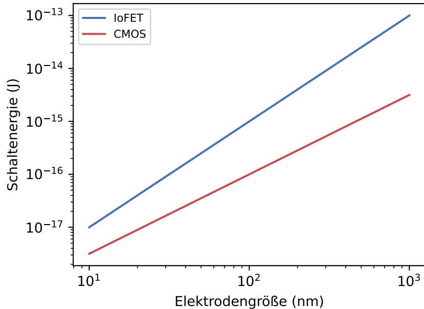
Schaltenergie vs. Elektrodenlänge
