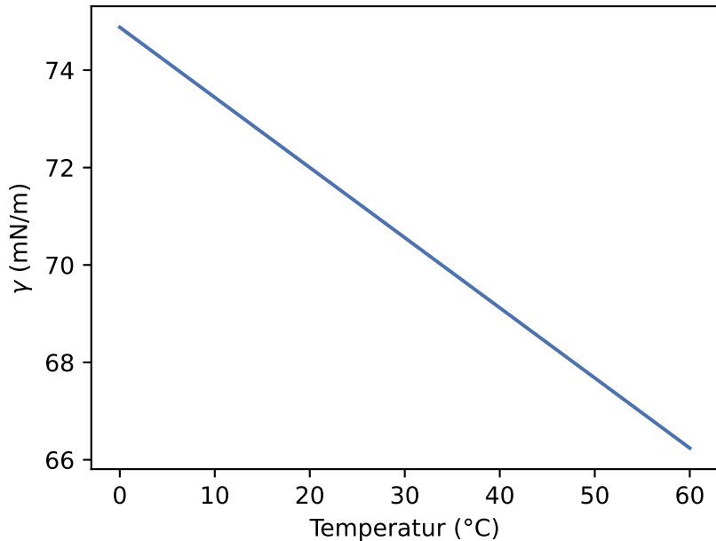
Oberflächenspannung vs. Temperatur
