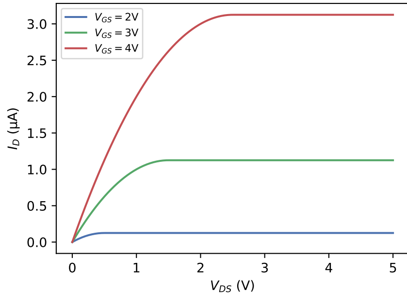
Ausgangskennlinienfeld
