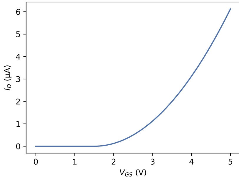
Transferkennlinie
