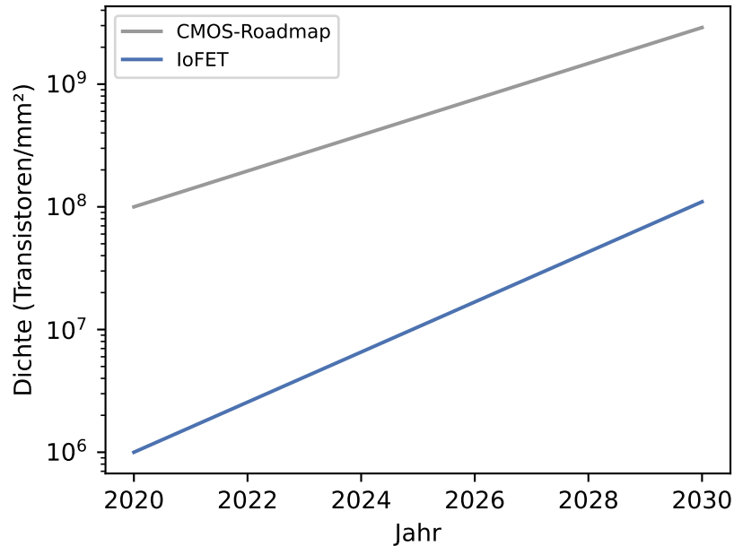
Transistordichte-Trend
