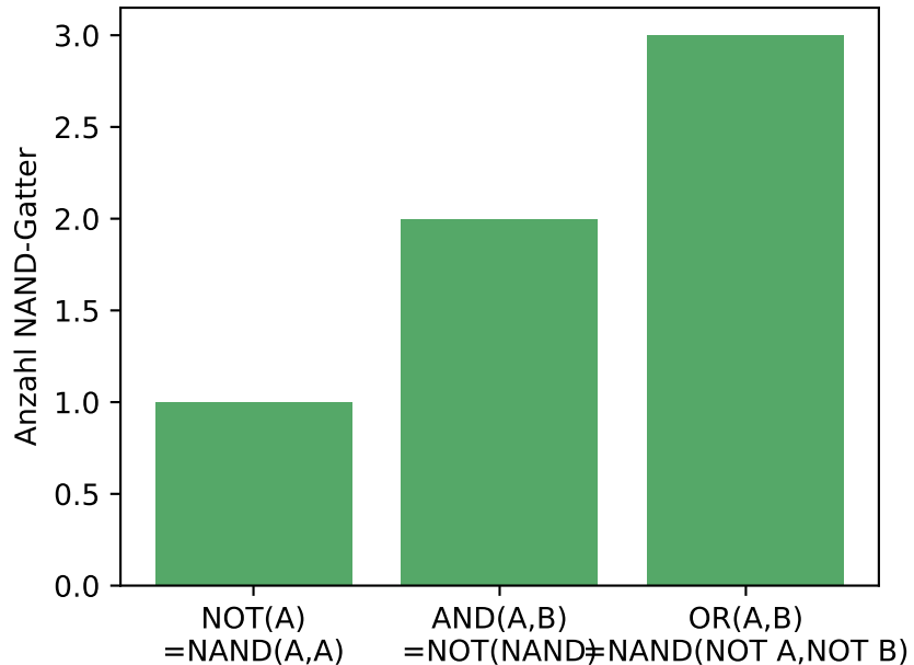
NAND-Vollständigkeit
