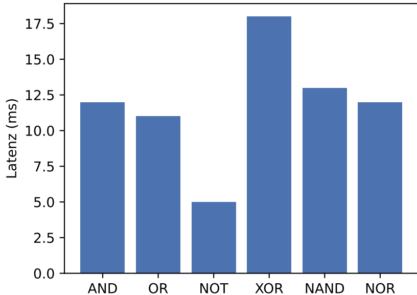
Logik-Gatter-Benchmark (Tropfen-Op.)
