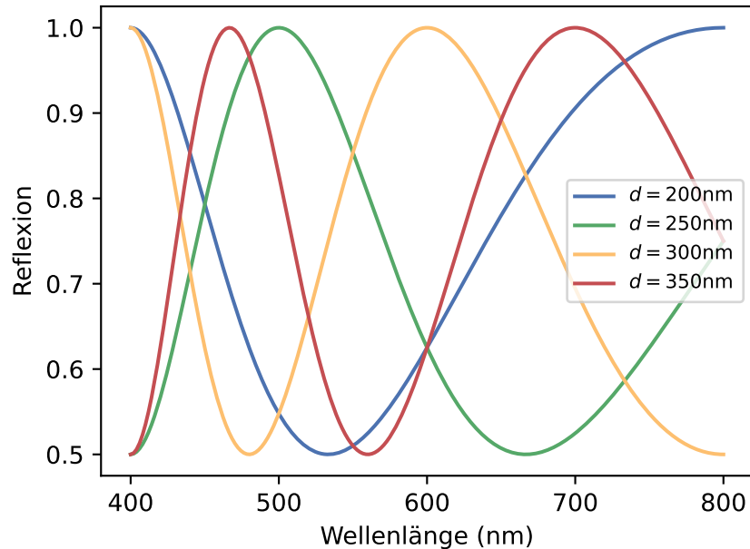
FP-Reflexionsspektren
