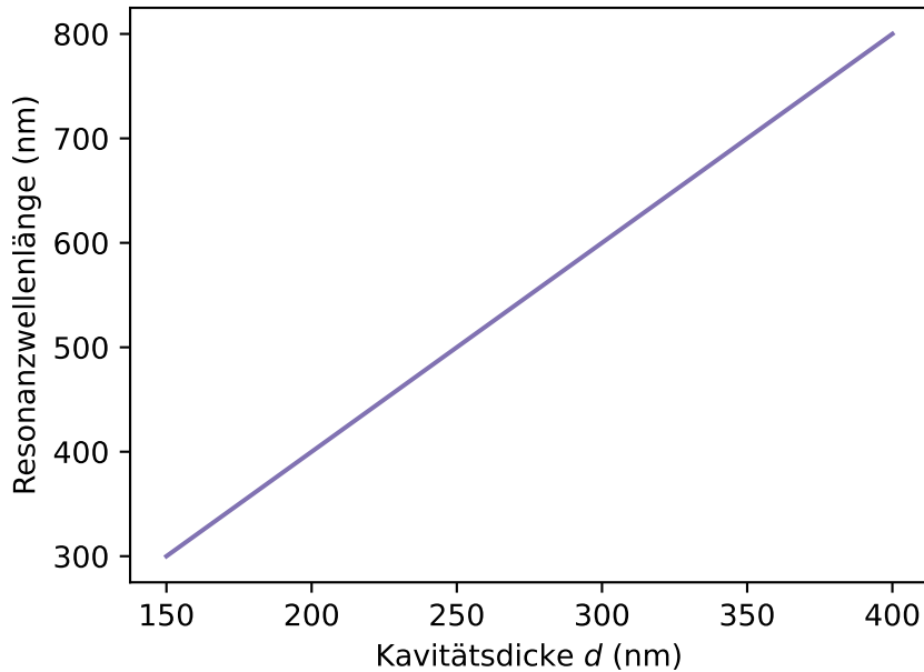
Farbdurchstimmbarkeit
