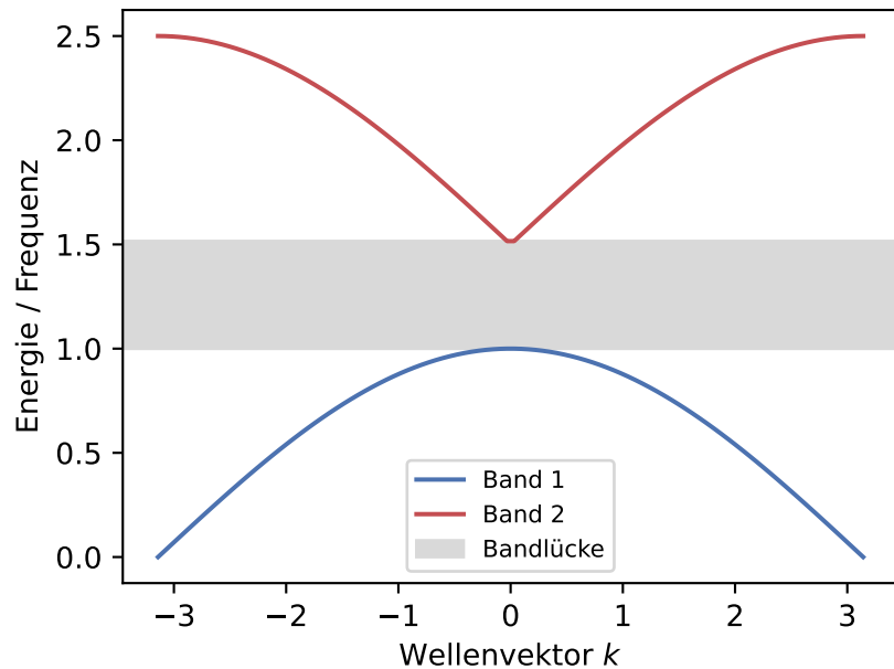
Photonische Bandstruktur
