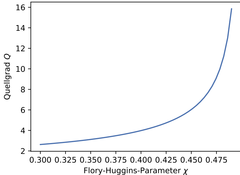
Flory-Rehner-Gleichgewichtsquellung
