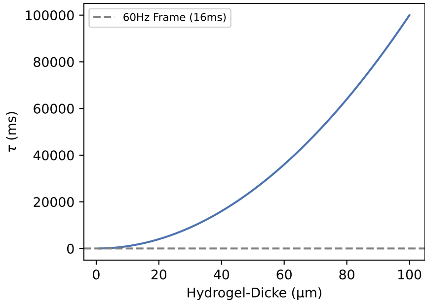
Quellungs-Relaxationszeit
