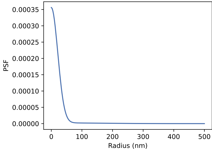
Chang-PSF (Punkt-Spread-Funktion)
