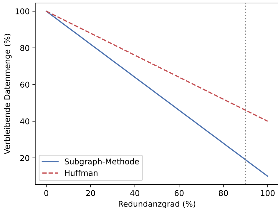
Komprimierungsrate vs. Redundanz
