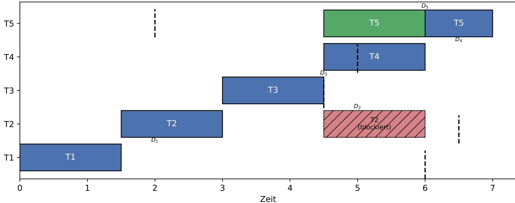
EDF + -Schedule mit Blocking und Neuplanung
