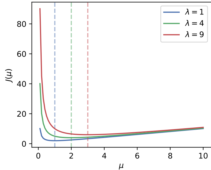
Kostenfunktional ( \mu^* = \sqrt{\lambda} )
