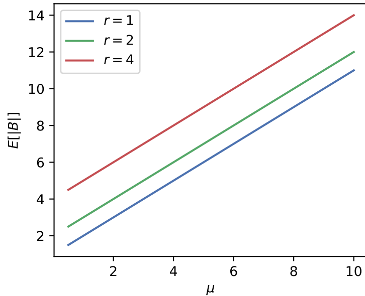
Erwartete Batchgröße (NegBin)
