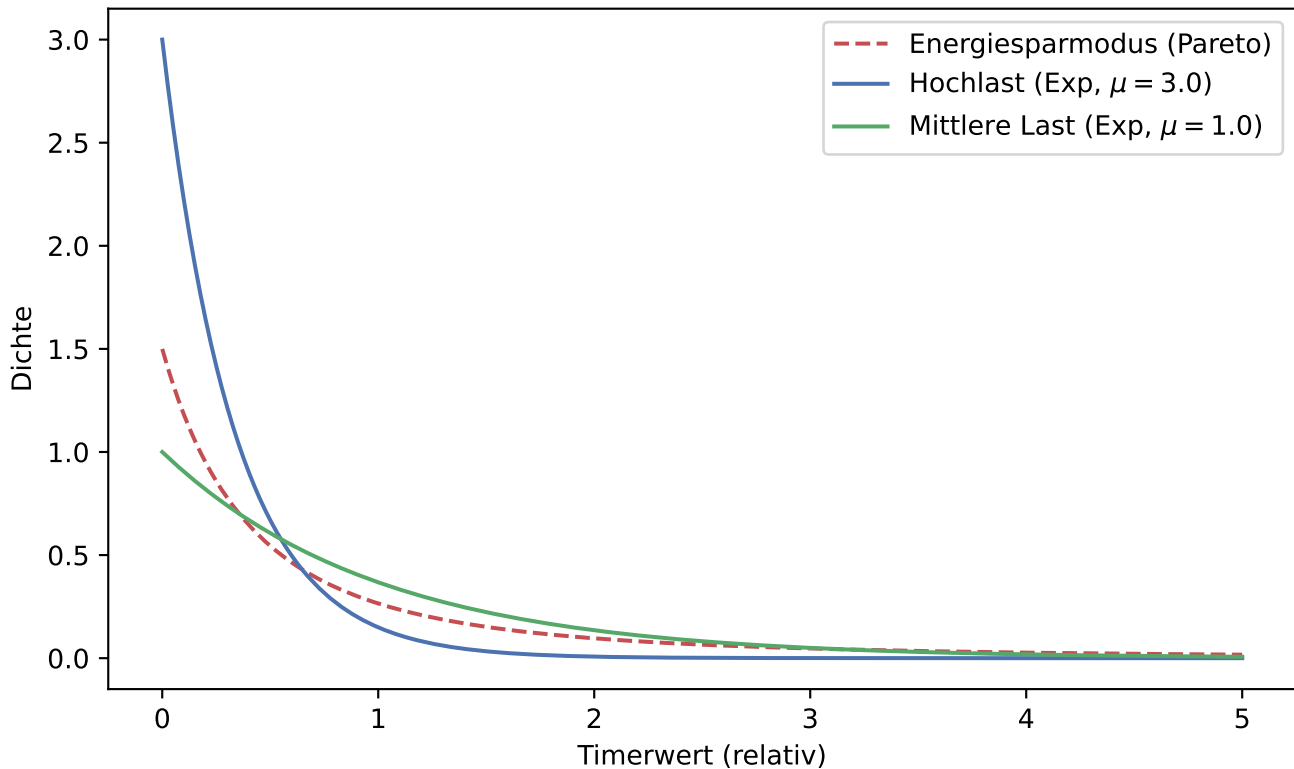
Timer-Dichtefunktionen für drei Lastregime
