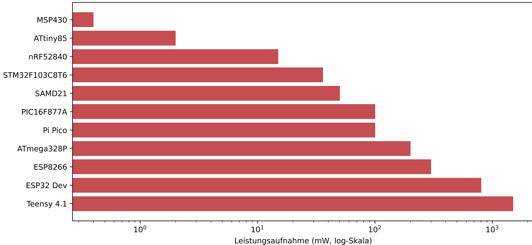
Typische Leistungsaufnahme im Aktivbetrieb
