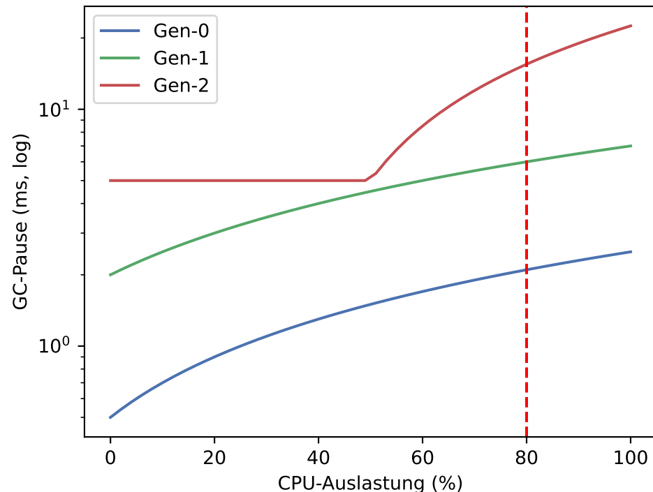
GC-Pausezeiten je Generation
