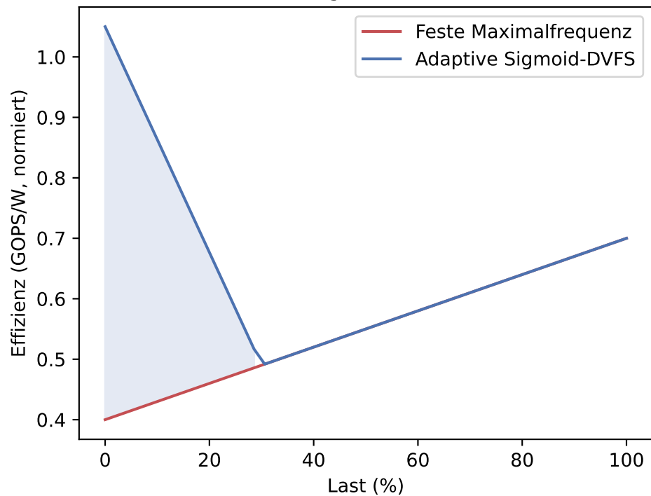
Energieeffizienz
