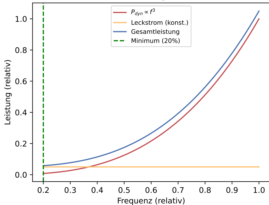
DVFS-Leistungsmodell
