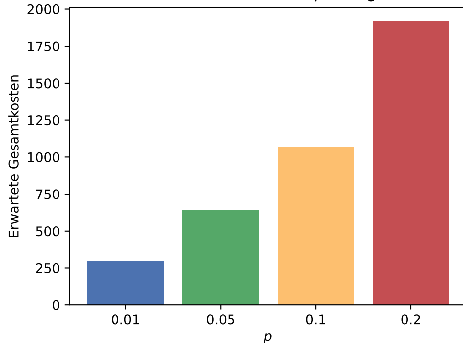
Gesamtkosten (1 + Np) \cdot n \log n
