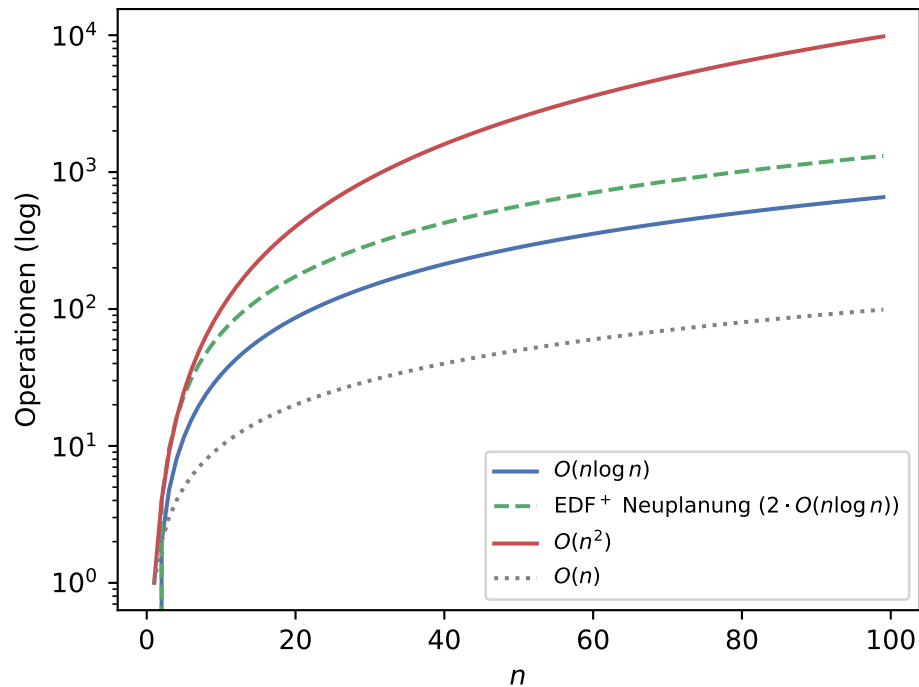
Laufzeitvergleich
