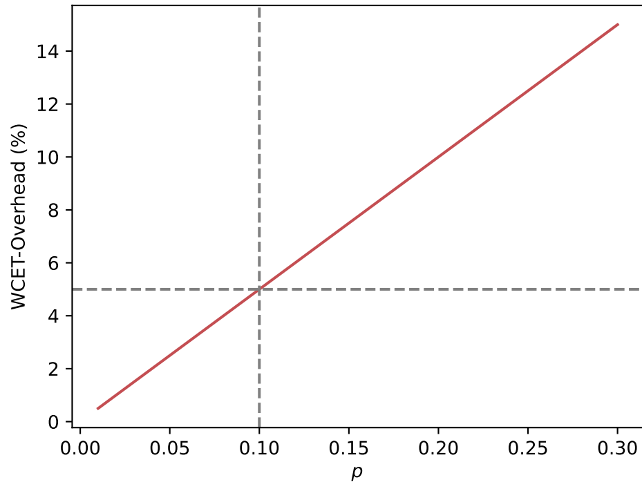
Normierter WCET-Overhead
