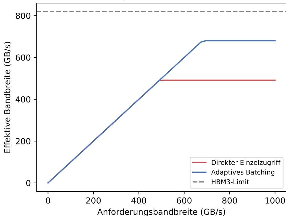
Effektive Speicherbandbreite (+38%)
