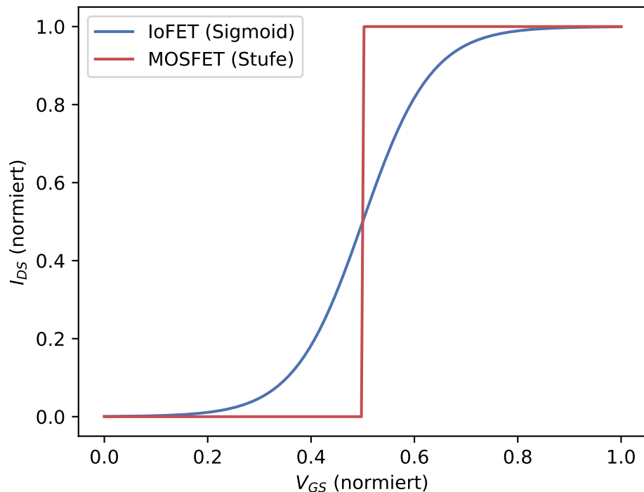
Transfercharakteristik IoFET vs. MOSFET
