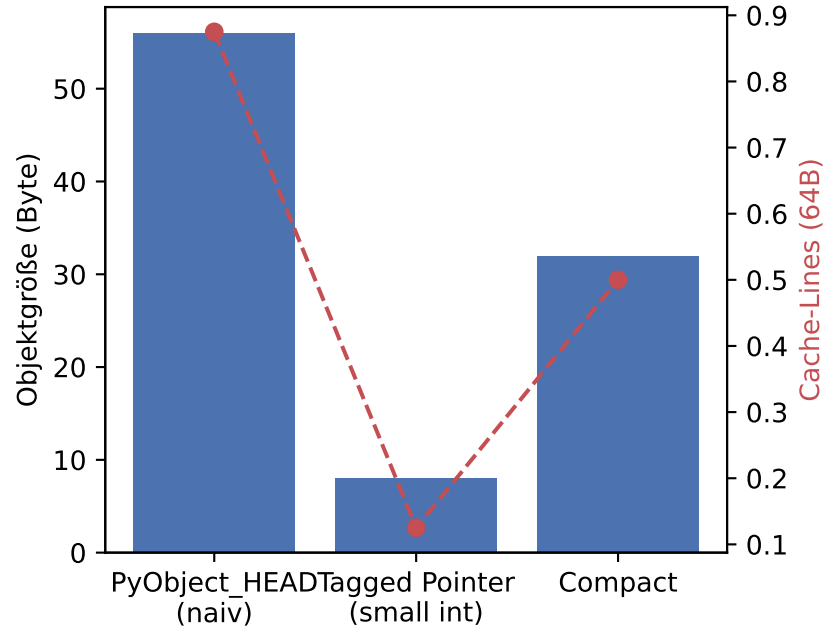
Python-Objektgrößen
