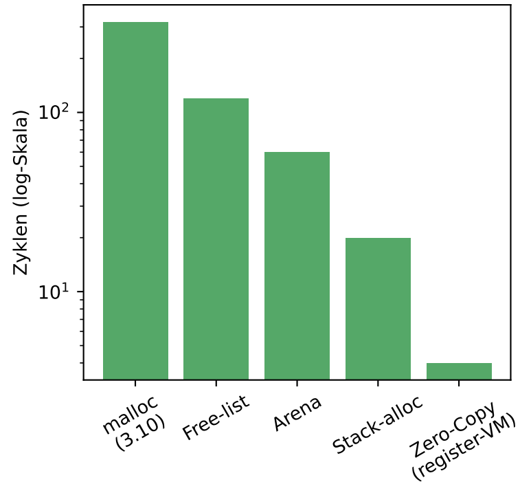
Frame-Allokations-Overhead
