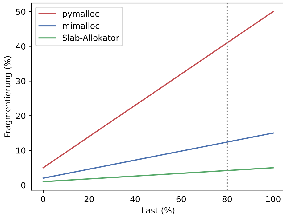
Fragmentierung bei steigender Last
