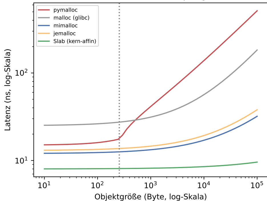
Allokationslatenz vs. Objektgröße
