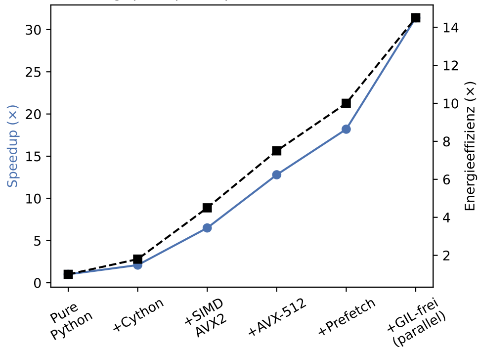
Throughput-Speedup auf PYMCA-8 (8 Kerne)
