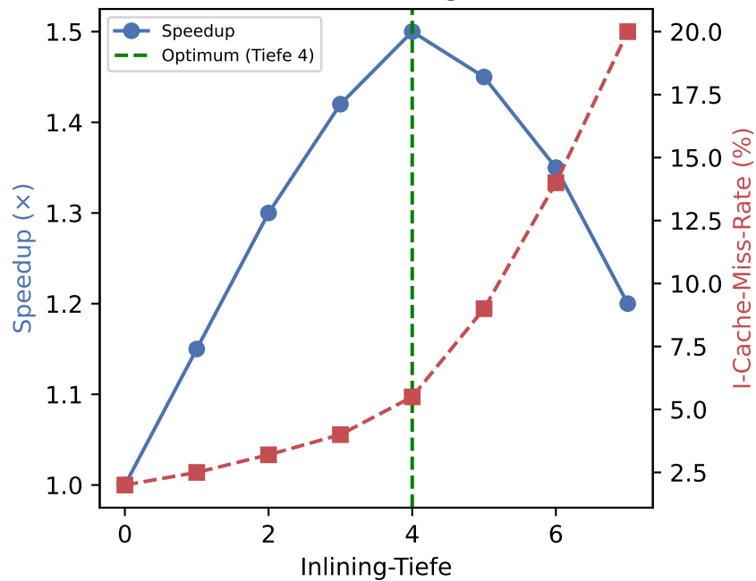
PGO/LTO: Inlining-Tiefe
