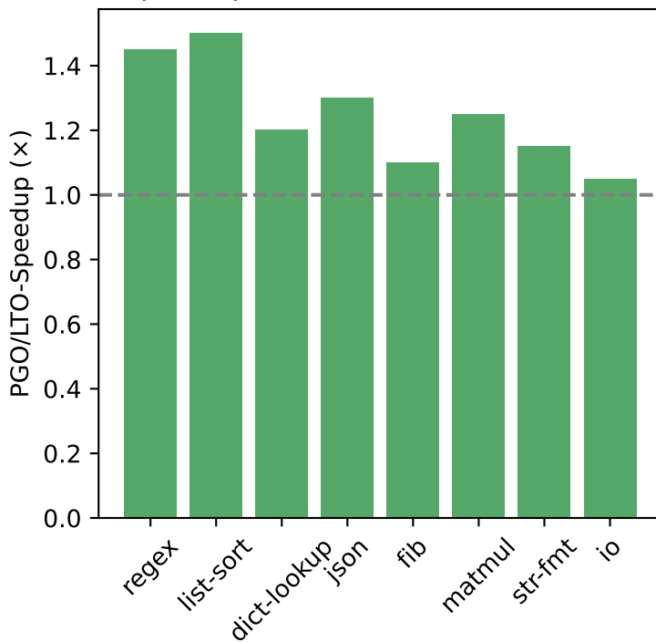
Speedup auf Standard-Benchmarks
