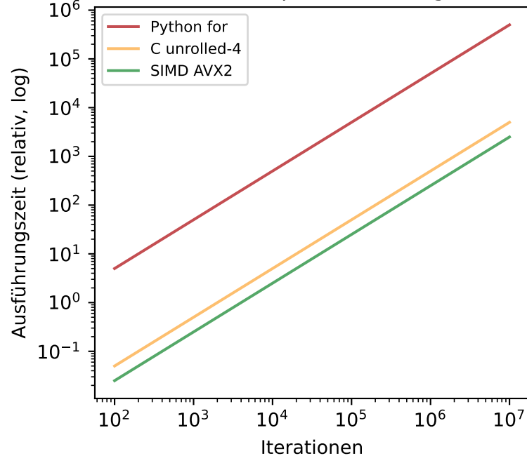
Schleifenimplementierungen
