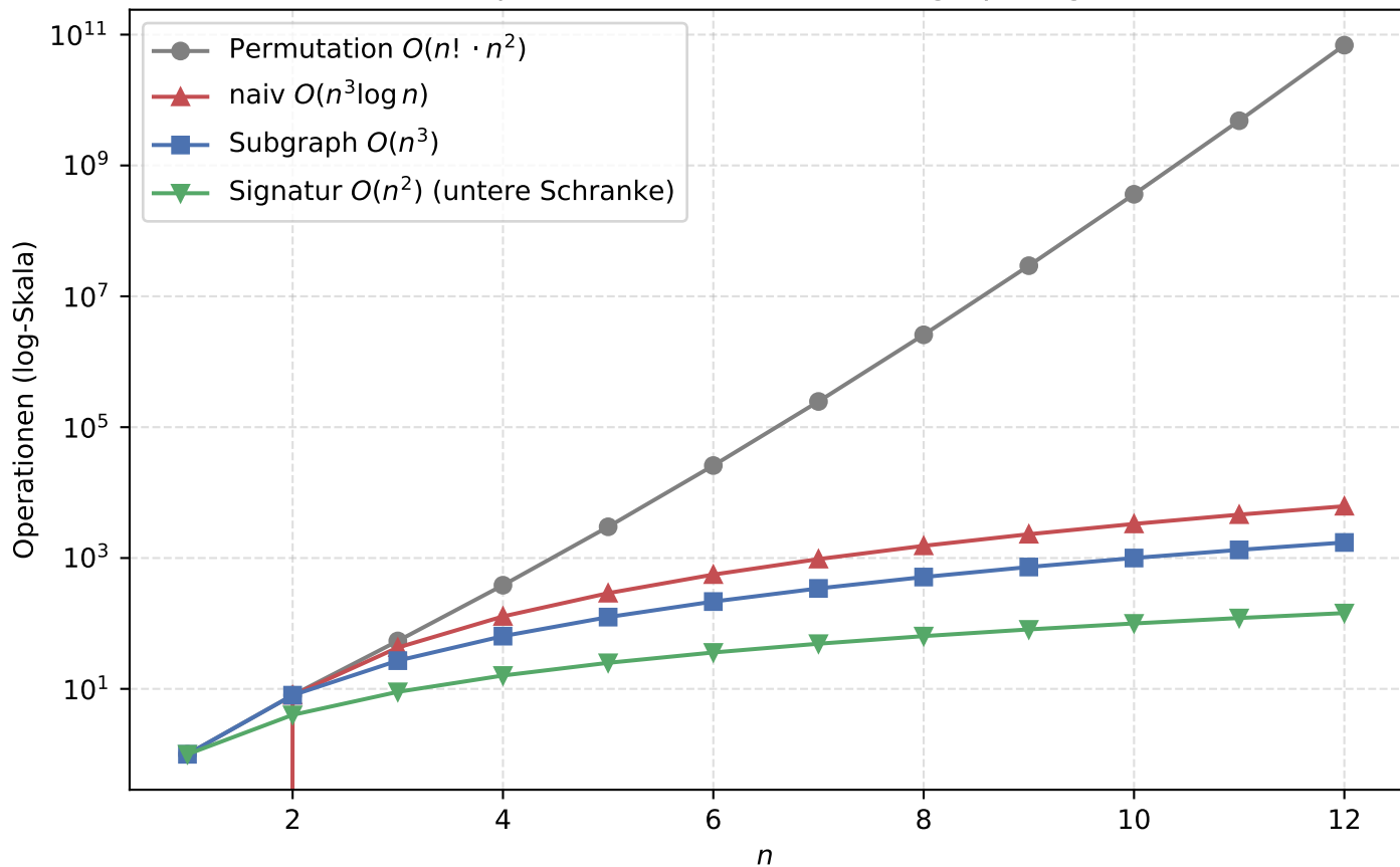
Laufzeitkomplexität verschiedener Subgraph-Algorithmen
