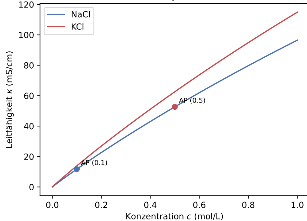
Ionische Leitfähigkeit (Kohlrausch)
