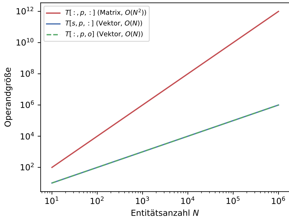
Tensor-Operandgröße
