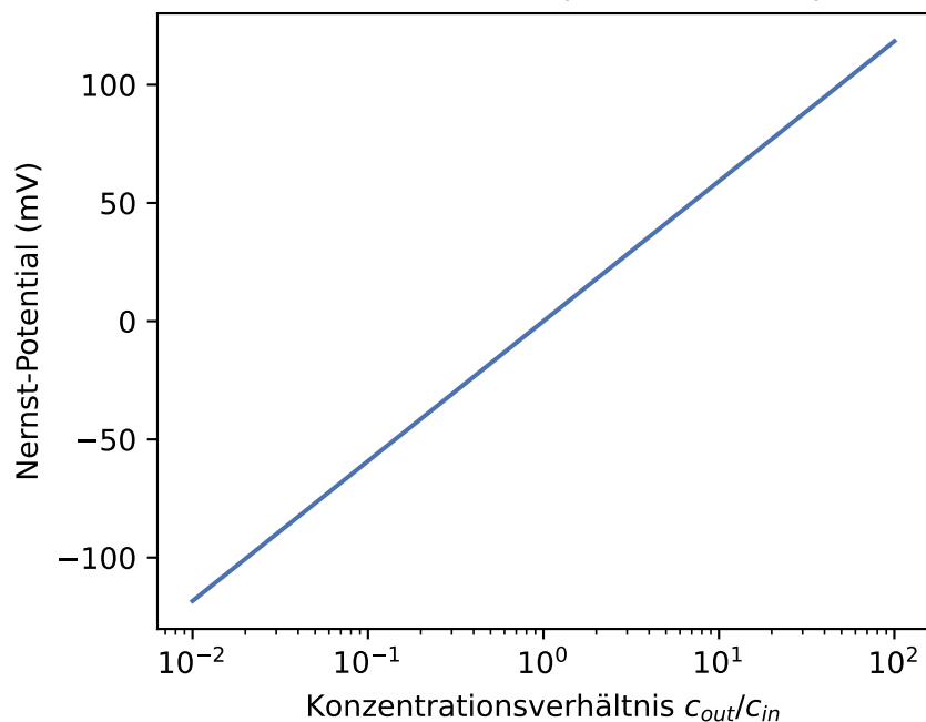
Nernst-Potential (kontinuierlich)
