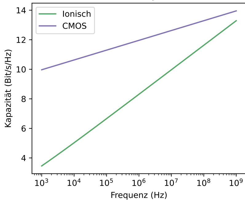
Shannon-Kapazität
