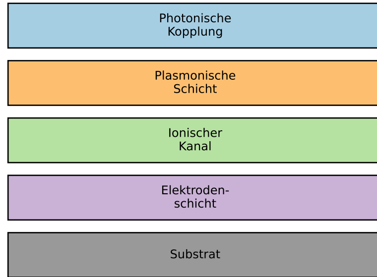
Fünfschichtige ionoxoqantum-Architektur
