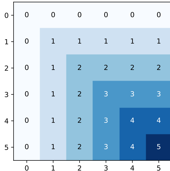
DP-Tabelle bester Rotation ( r = 0 )
