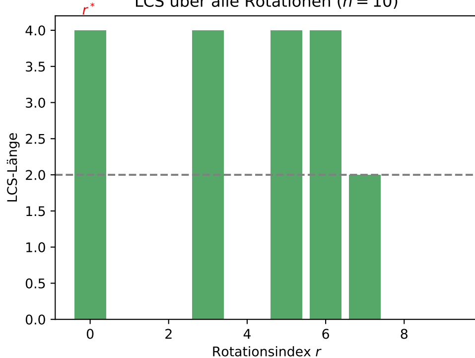
LCS über alle Rotationen ( n = 10 )
