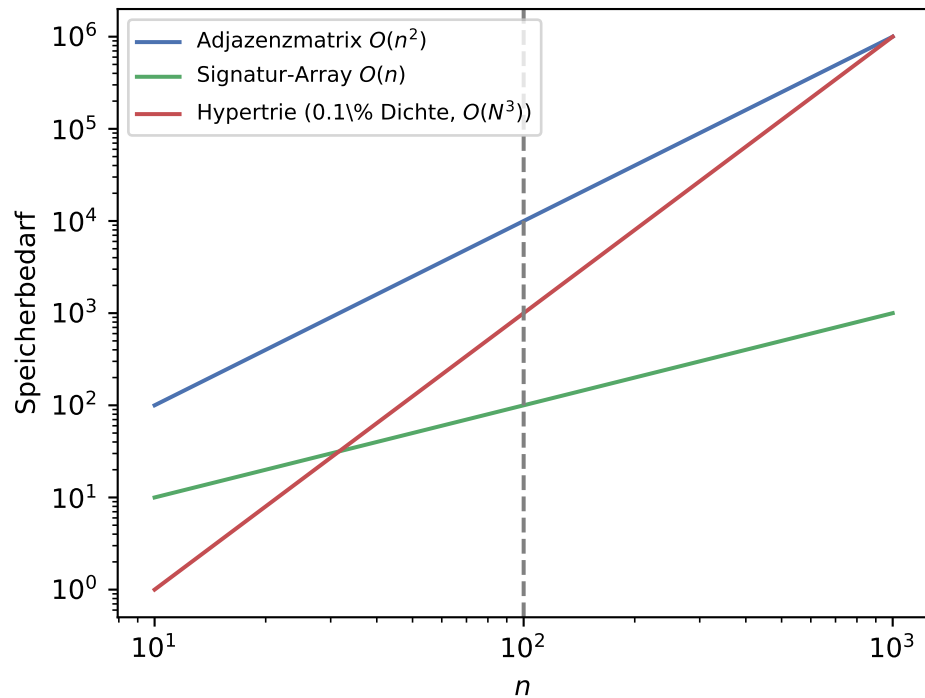
Speicherbedarf-Vergleich
