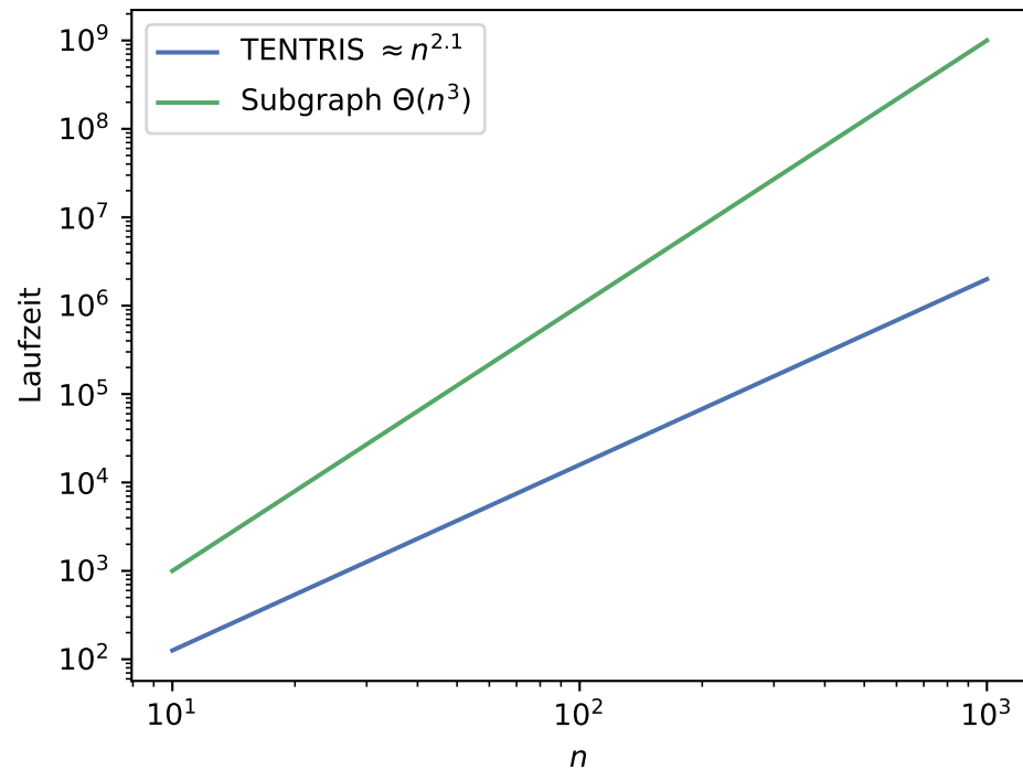
Skalierungsvergleich
