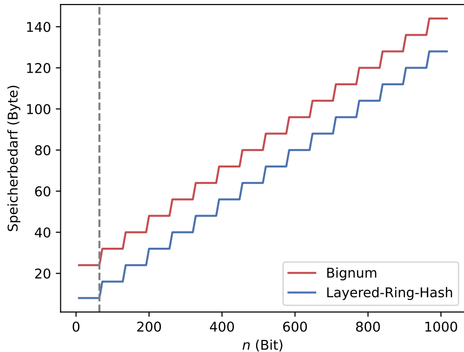
Speicherbedarf: Bignum vs. LRH
