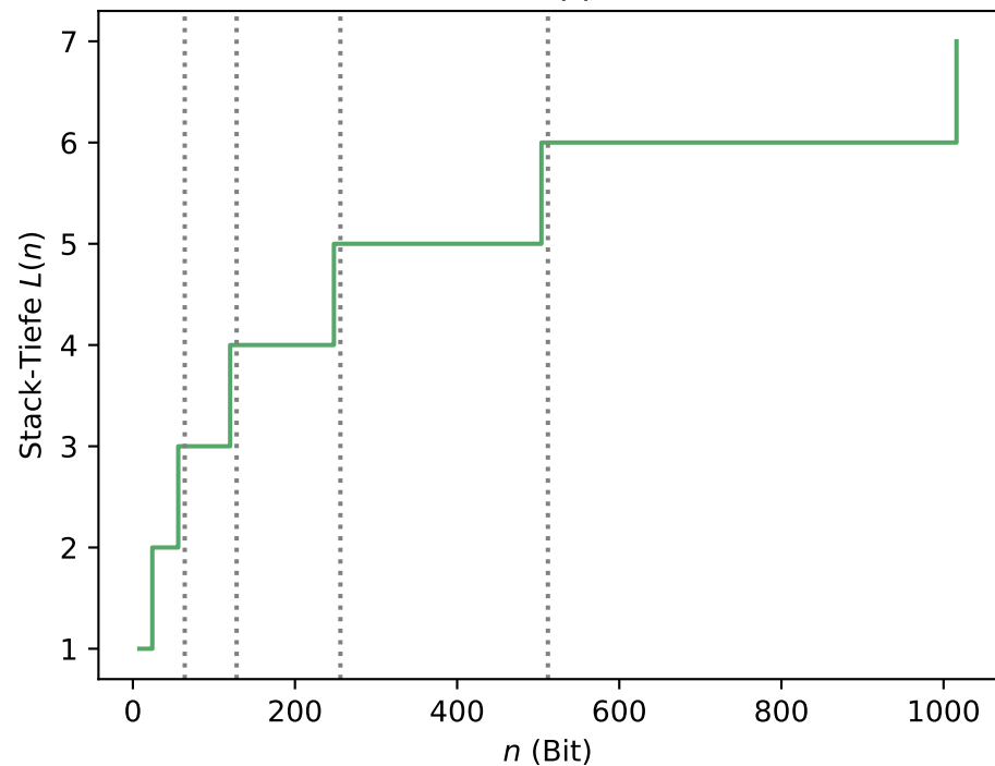
Stack-Tiefe (Treppenfunktion)
