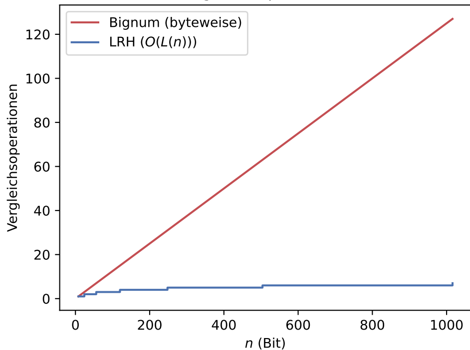
Vergleichsoperationen
