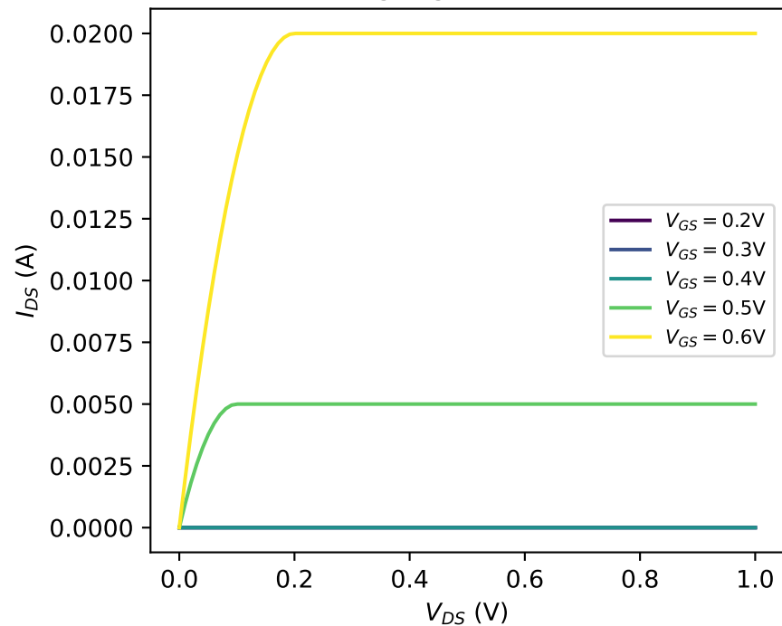
Ausgangskennlinien
