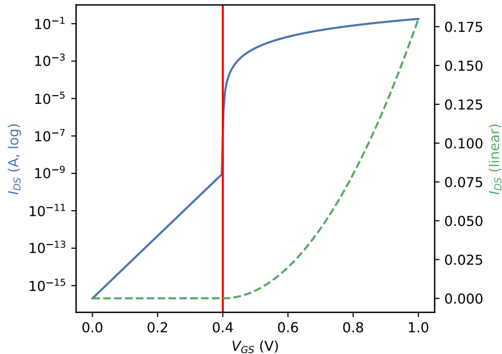
Übertragungskennlinie ( V_{DS} = 50\text{mV} )
