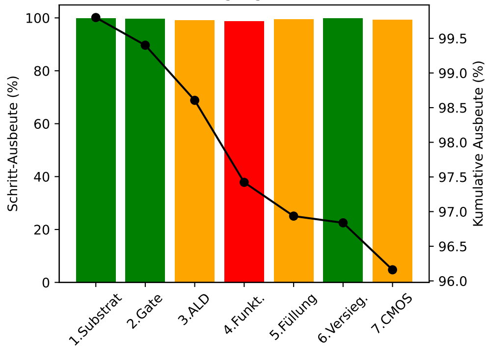
IRF-1 Fertigungsausbeute
