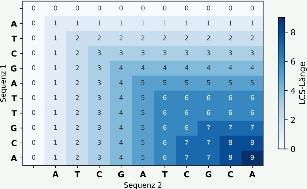
Sequenzalignment als LCS-DP |LCS| = 9 von \min(10, 10) = 10
