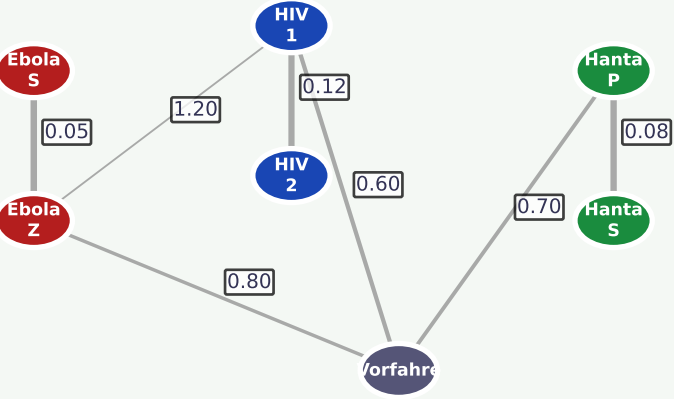
Phylogenetischer Graph G_{phylo} (Evolutionäre Distanzen als Kantengewichte)
