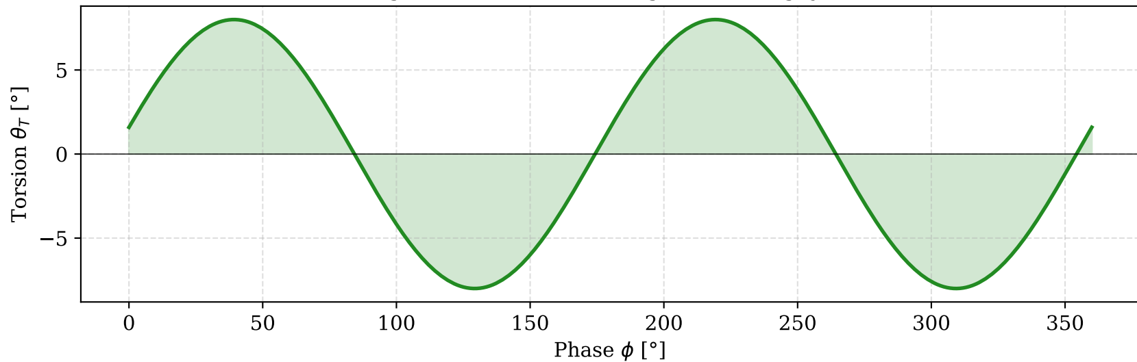
Flügeltorsion (Verdrillung) im Schlagzyklus
