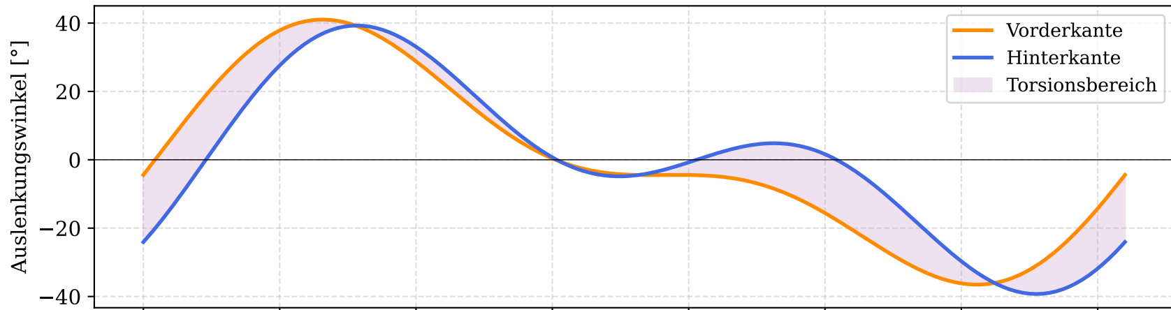
Flügelbewegungskinematik über einen Schlagzyklus ( T = 100 ms)
