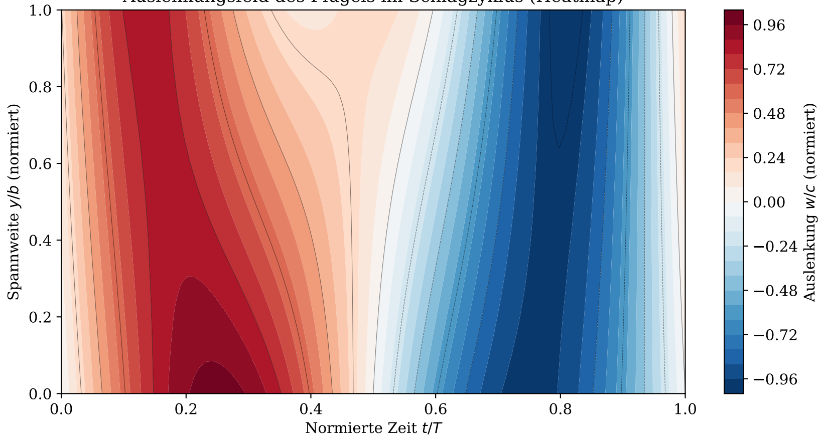
Auslenkungsfeld des Flügels im Schlagzyklus (Heatmap)
