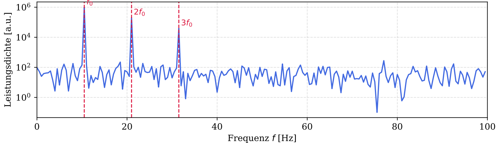
Leistungsspektrum des Flügelschlagsignals
