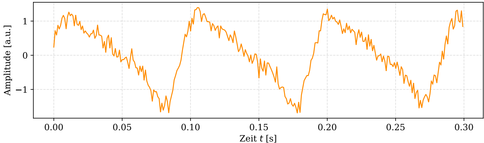
Beschleunigungssignal am Flügelwurzel (Vanessa atalanta)
