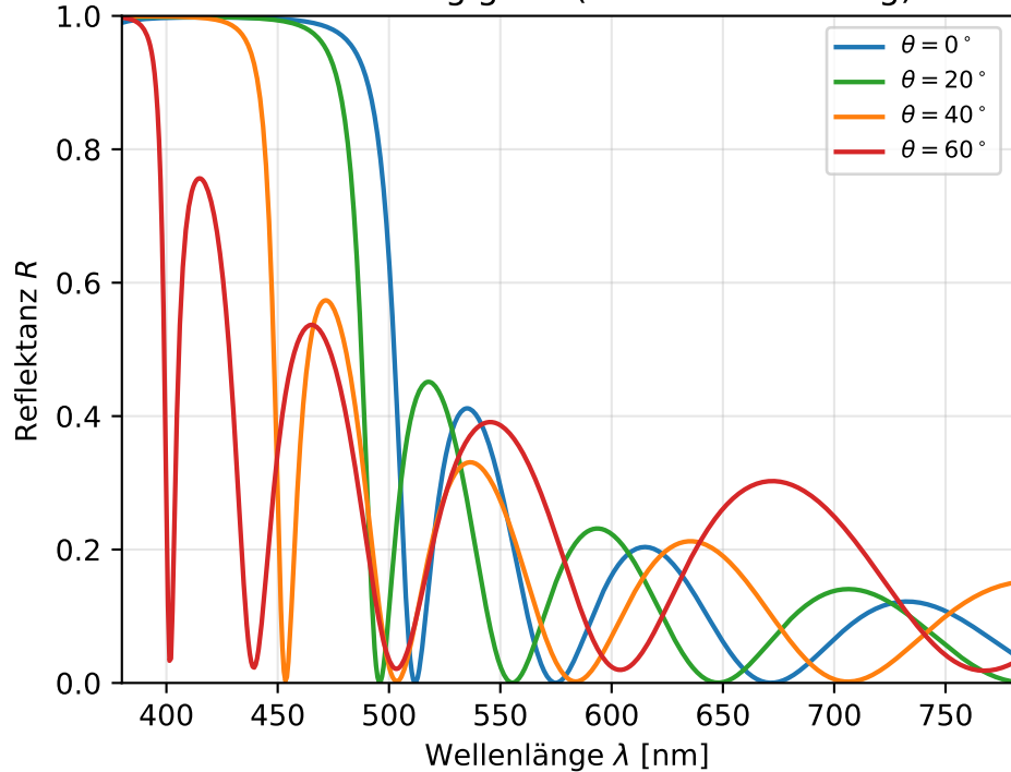
Winkelabhängigkeit (Blauverschiebung)
