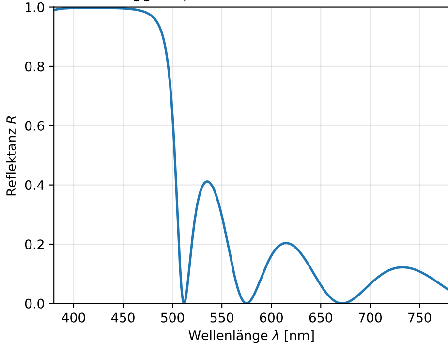
Bragg-Stapel ( N = 8 Perioden), \theta = 0^\circ
